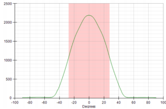
光強度(Candela)
